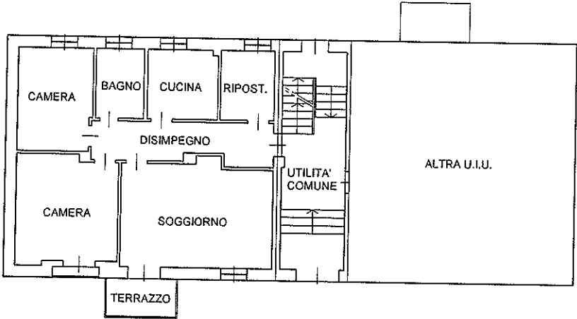
PIANO RIALZATO H= 2,77 m
