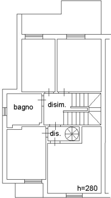
PIANO SECONDO
