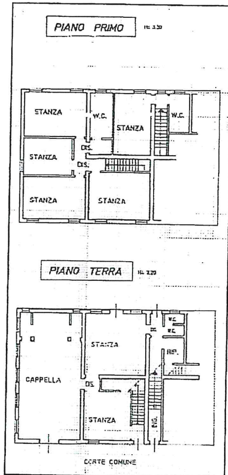
Planimetrie del Fabbricato 1
